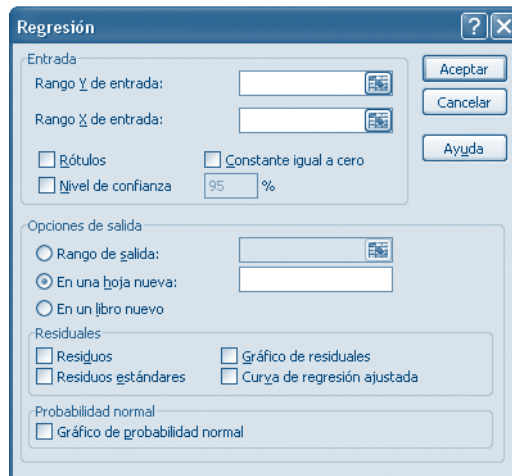
Figura 39. Regresión
